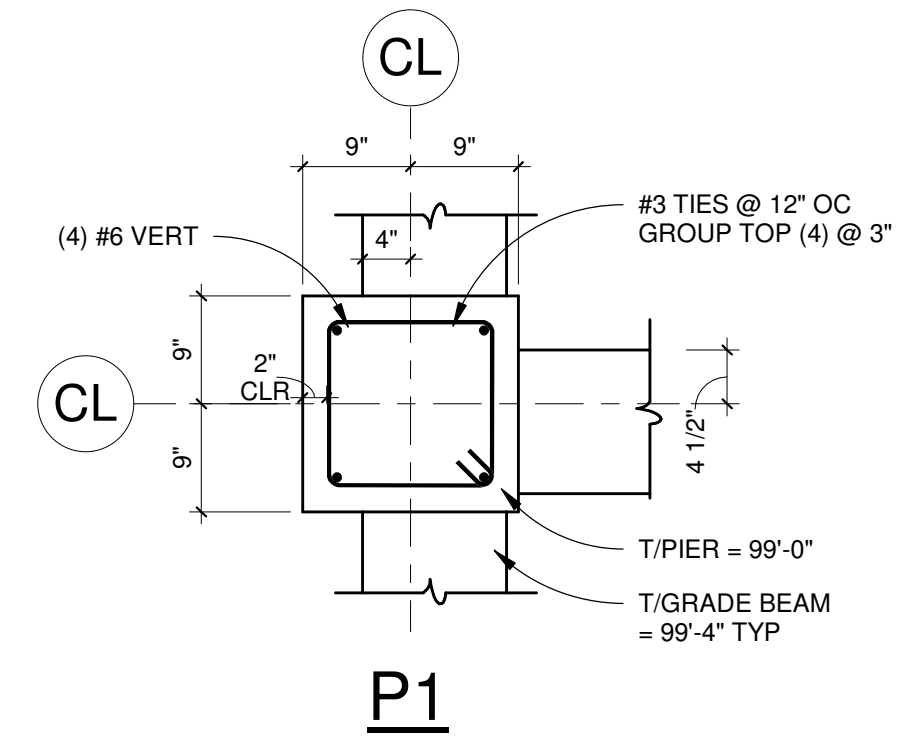
1 PIERS SCALE: 3/4" = 1'-0"
