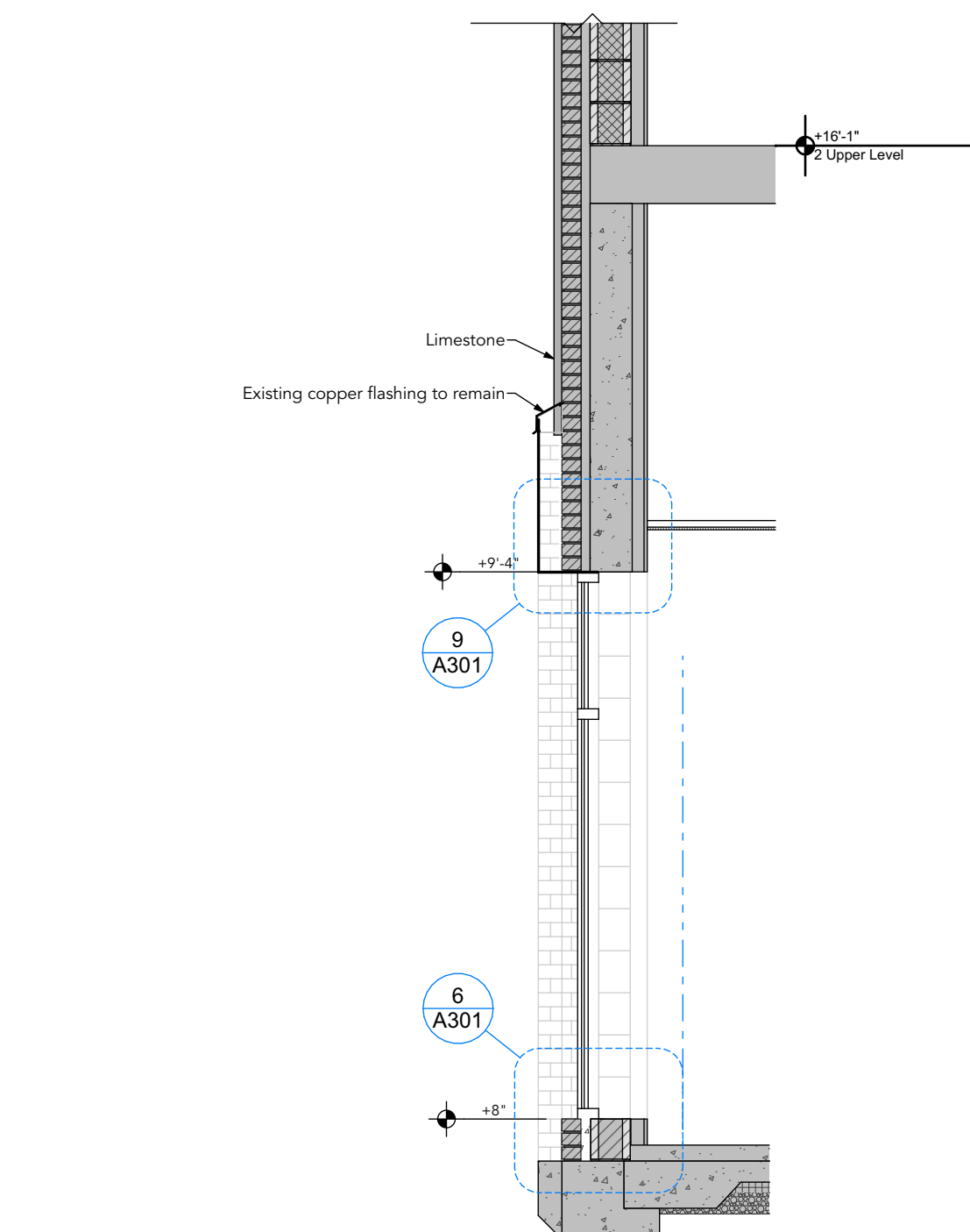
2 Storefront @ Concrete Header & Metal Panel A301 SCALE: 3/8" = 1'-0"
