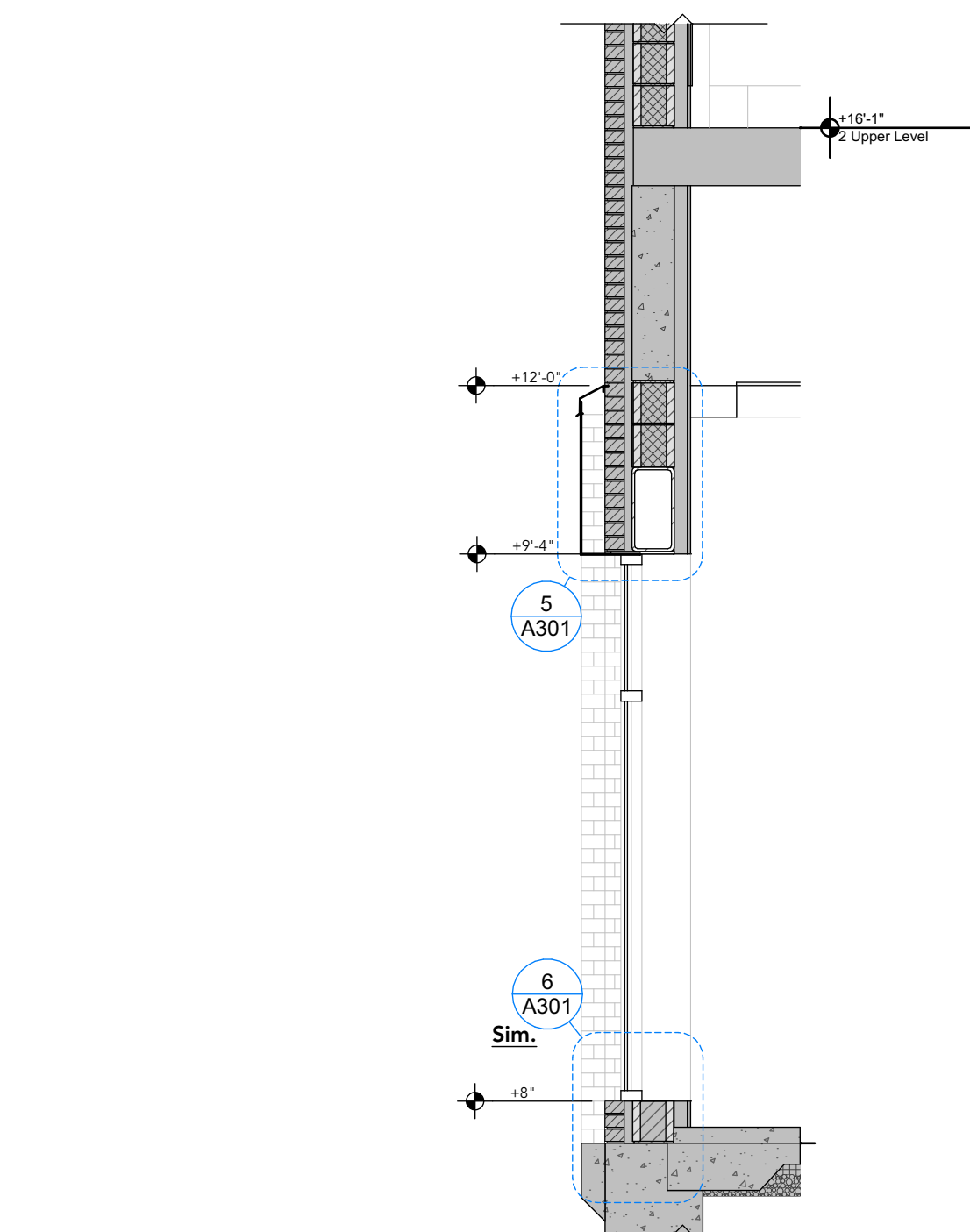
1 Storefront @ CMU Header & Metal Panel A301 SCALE: 3/8" = 1'-0"
