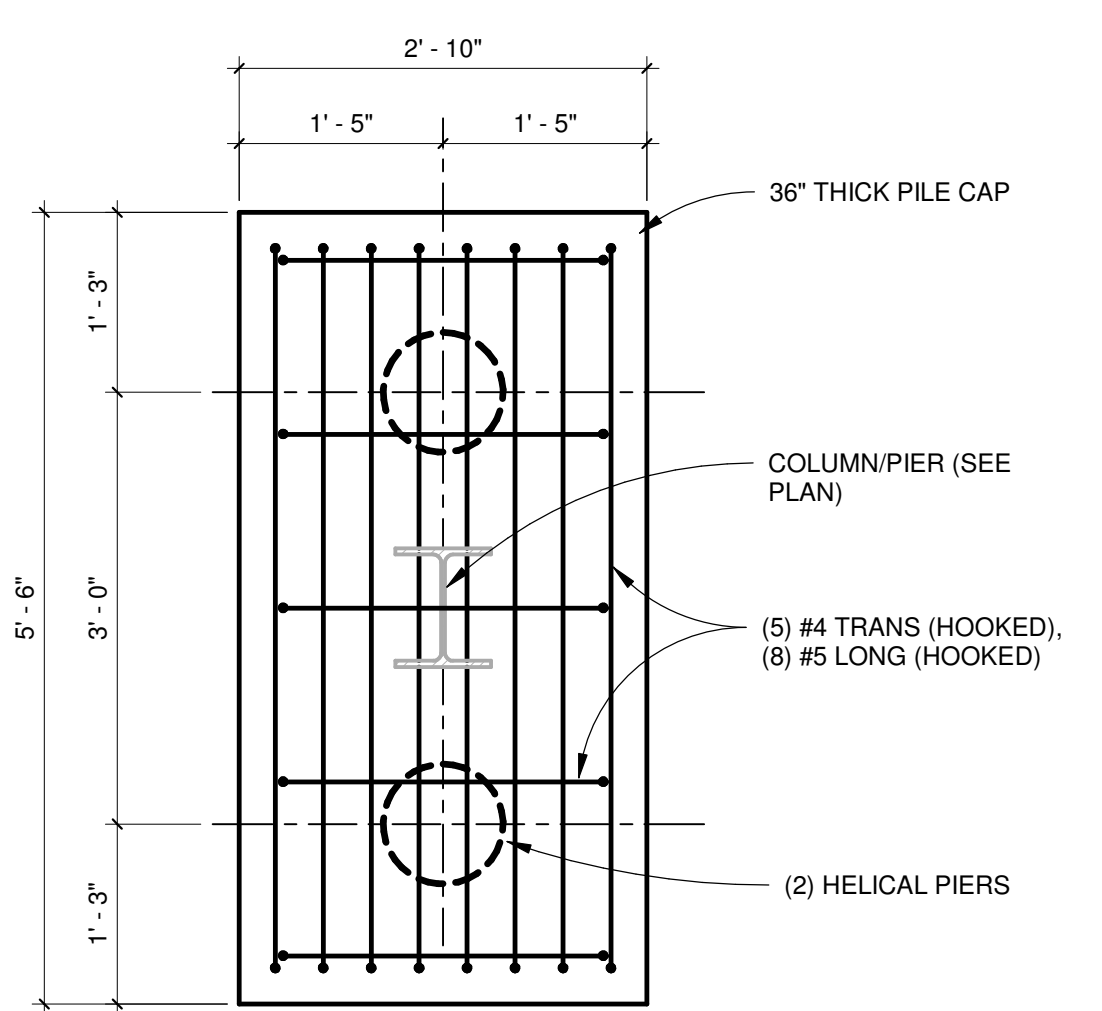
11 S201 PILE CAP PH2 SCALE: 3/4" = 1'-0"
