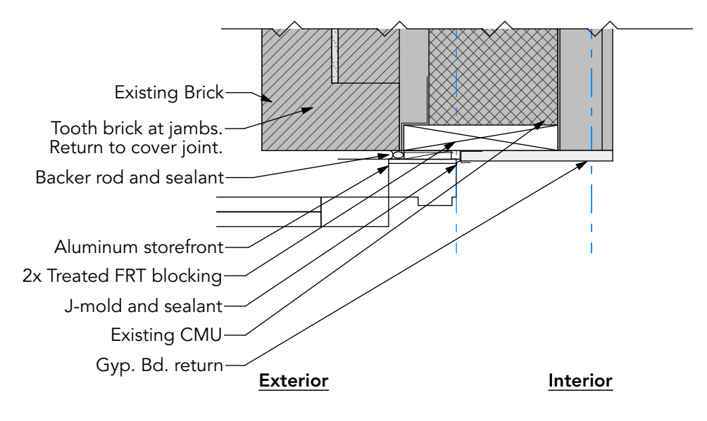
13 Aluminum SF Door Jamb A301 SCALE: 1 1/2" = 1'-0"
