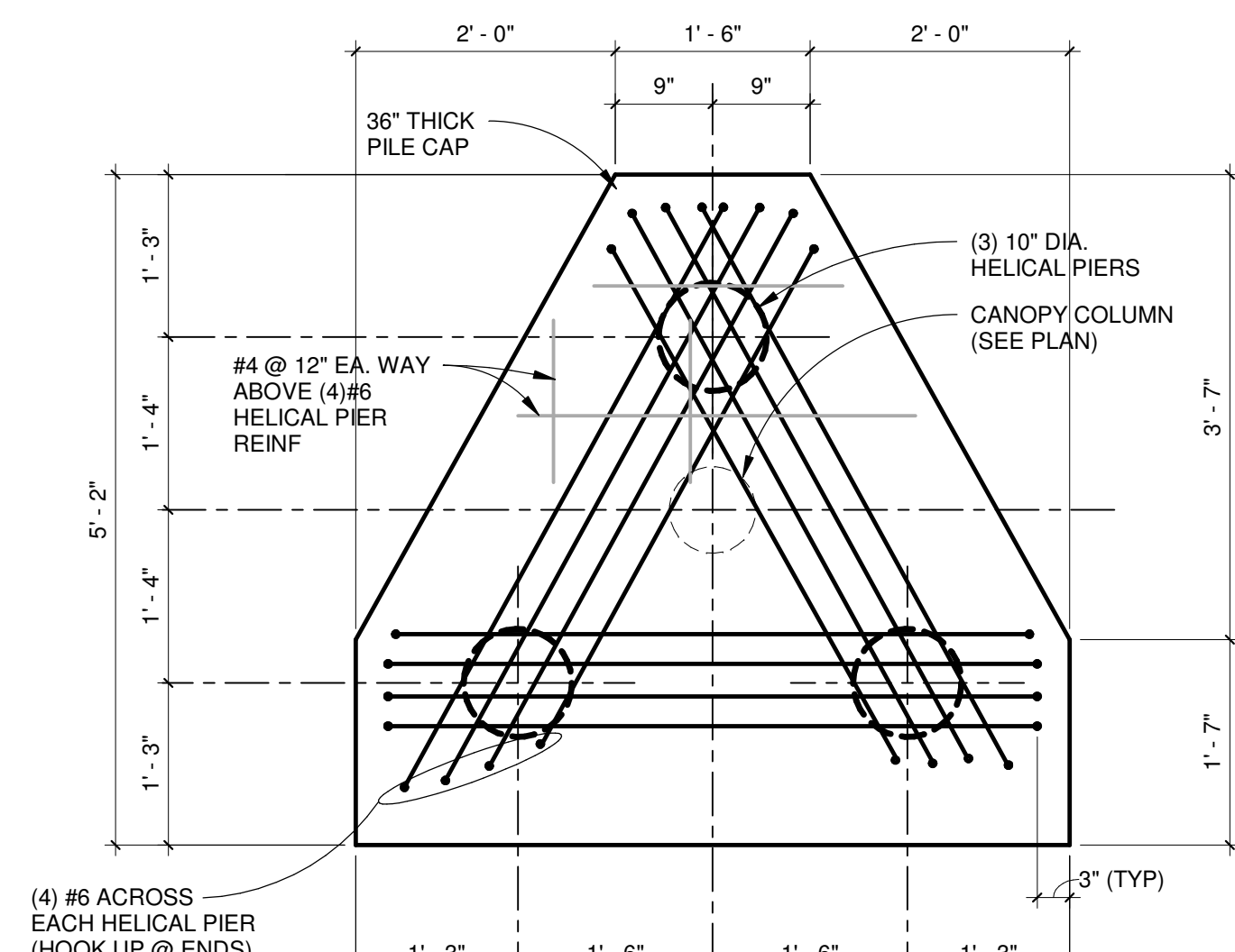
12 S201 PILE CAP PH3 SCALE: 3/4" = 1'-0"
