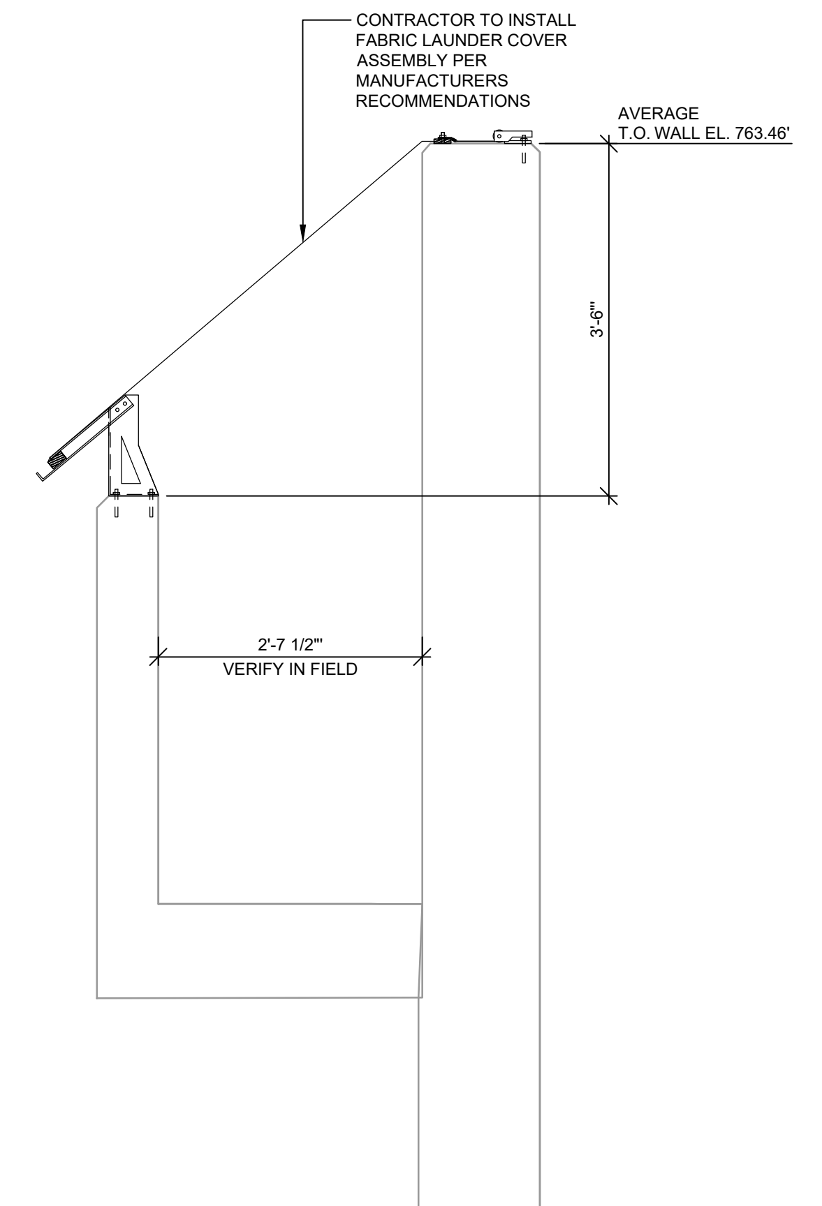
SECTION A-A SCALE: 3/4" = 1'-0"
